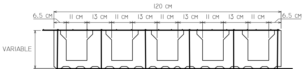
SECCIÓN A-A'
