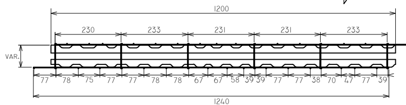
SECCION A-A'
